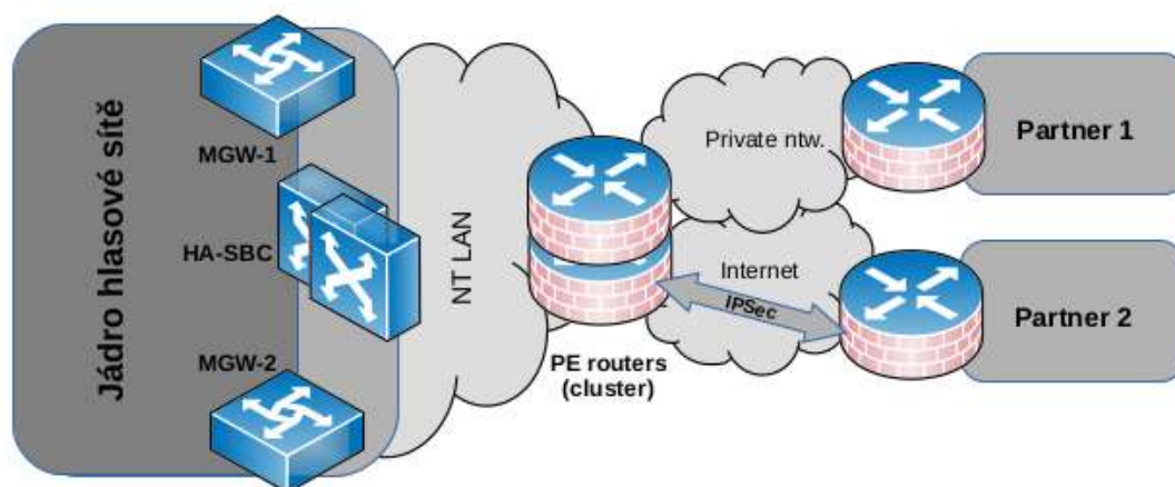
Obr.1 Obecná hierarchie propojení hlasové sítě
