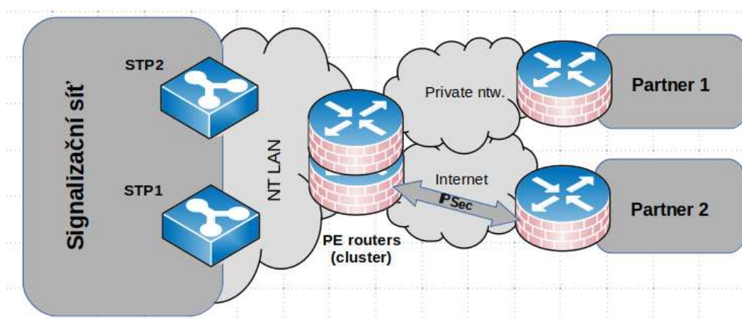
Obr.2 Obecná hierarchie propoje signální sítě
